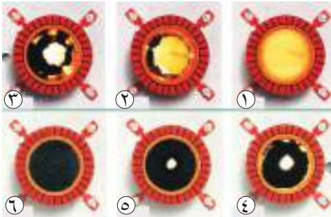
طریقه عملکرد حلقه ضد آتش در هنگام آتش‌سوزی
